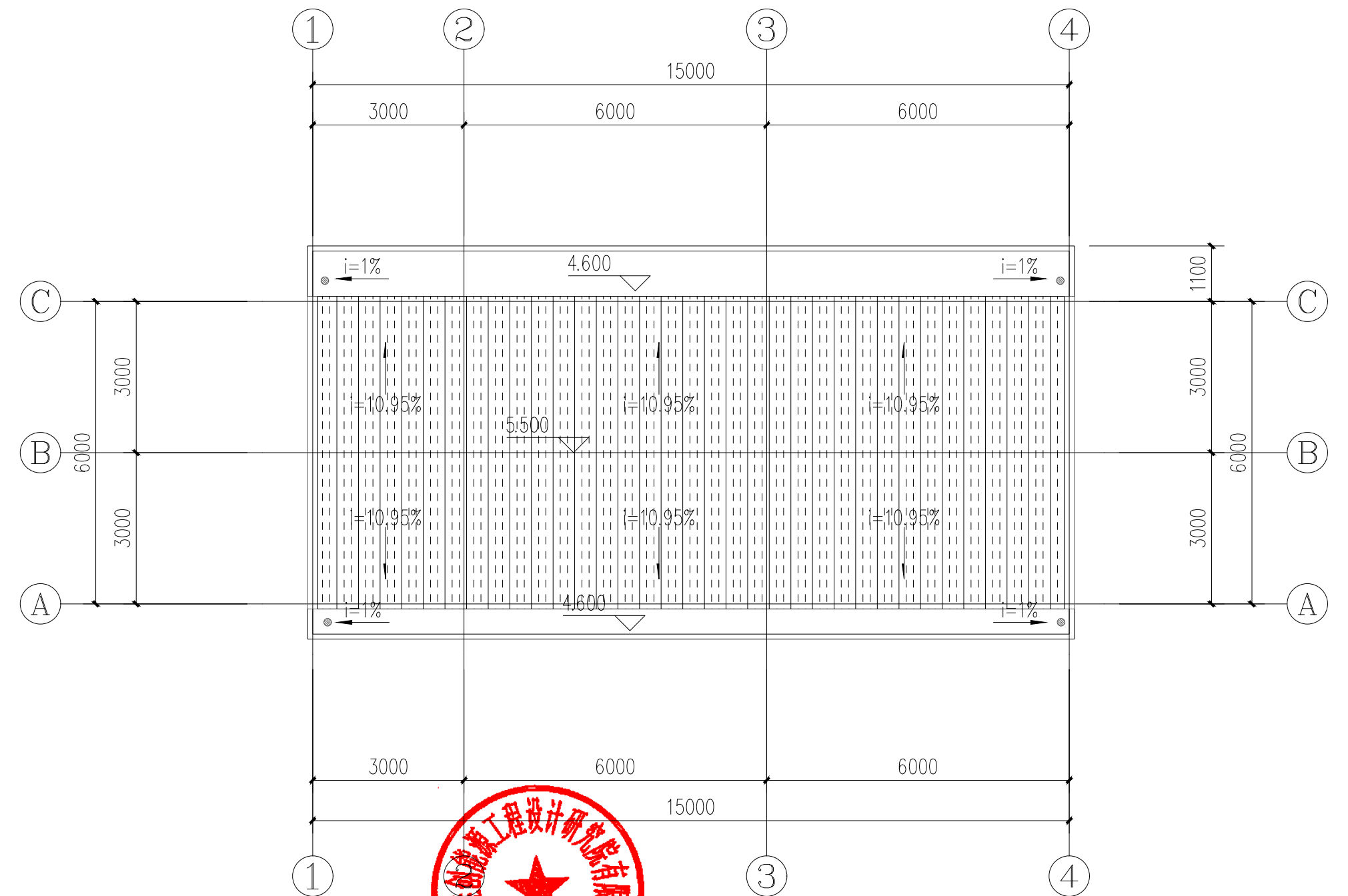
屋面平面图 1:100
