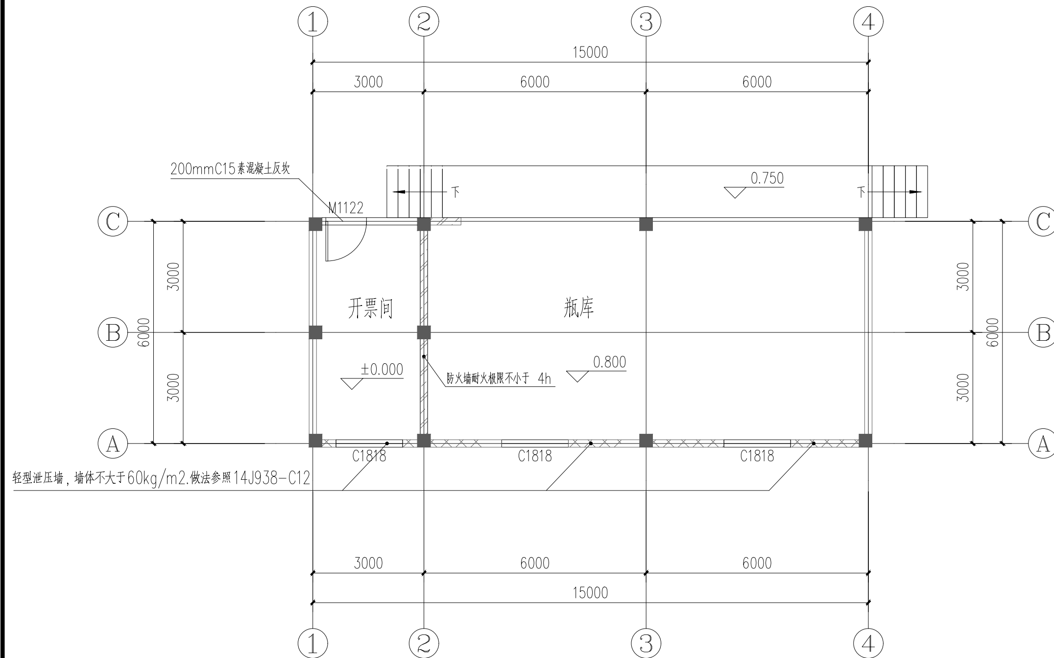
一层平面图 1:100
