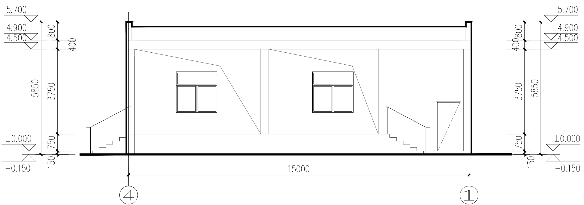
4~1 轴立面图 1:100
