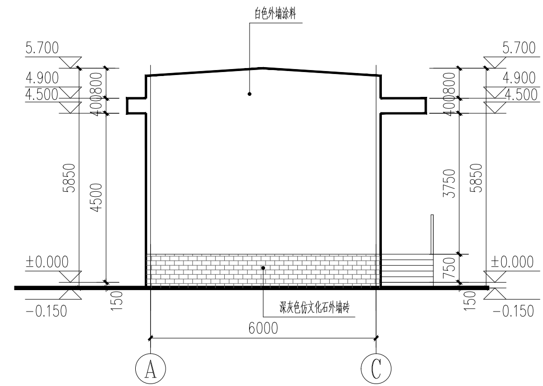
A~C 轴立面图 1:100
