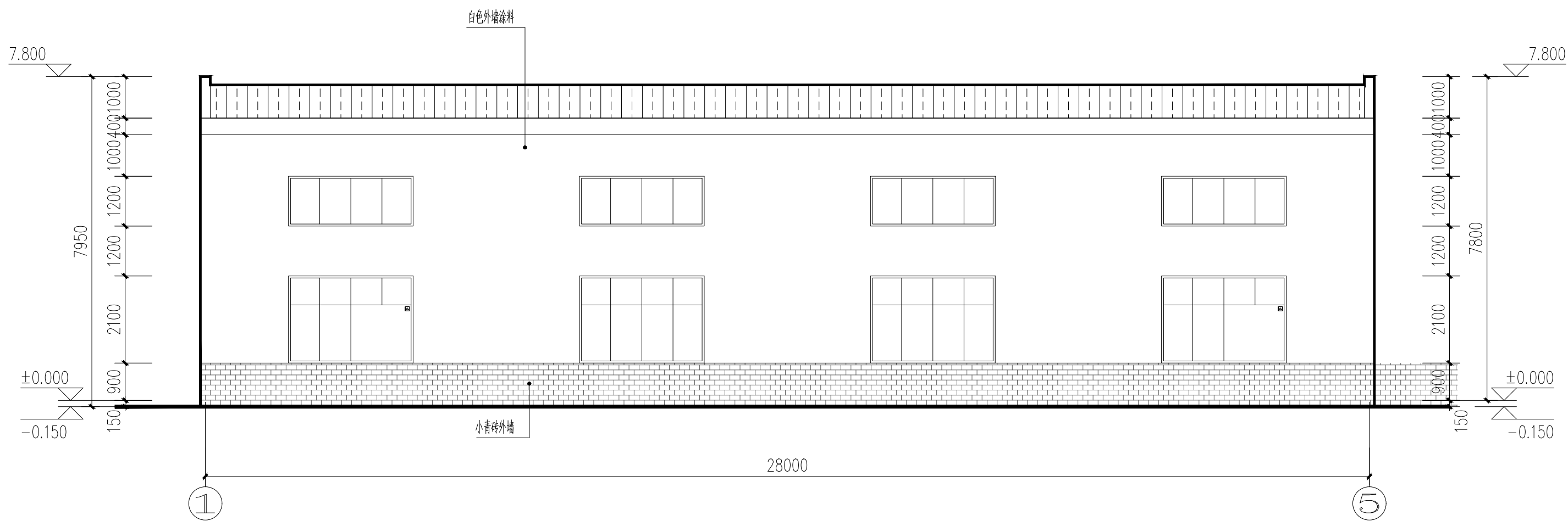
① ~ ⑤ 轴立面图
