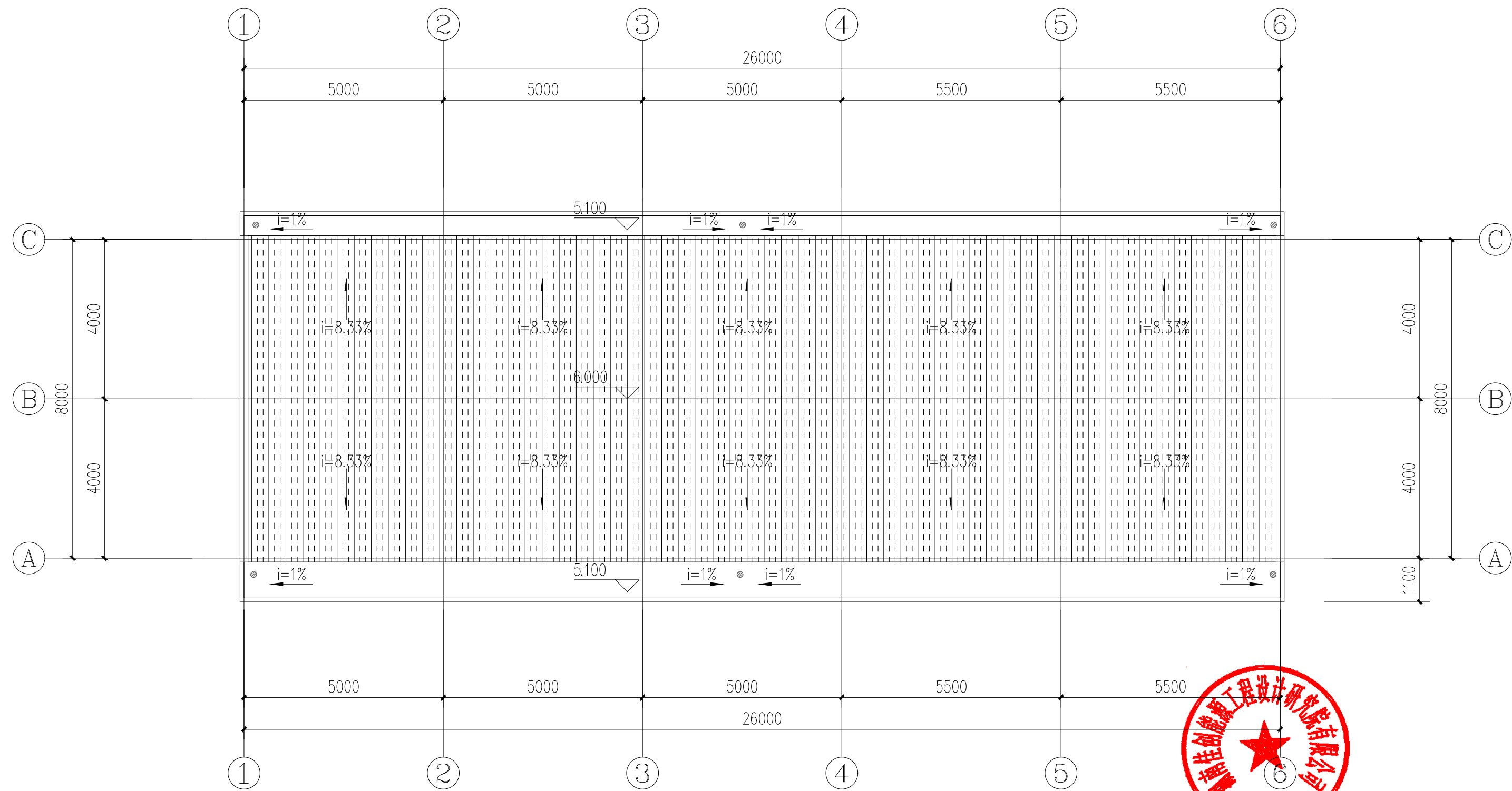
屋面平面图 1:100
