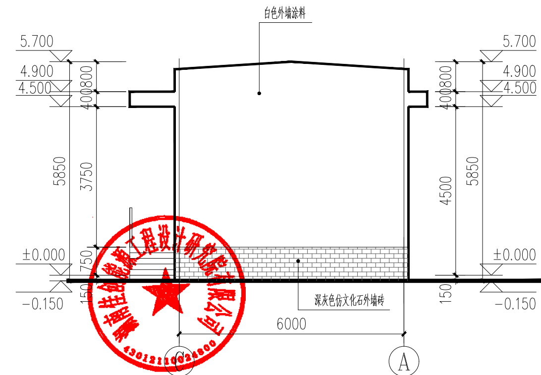
C~A 轴立面图 1:100
