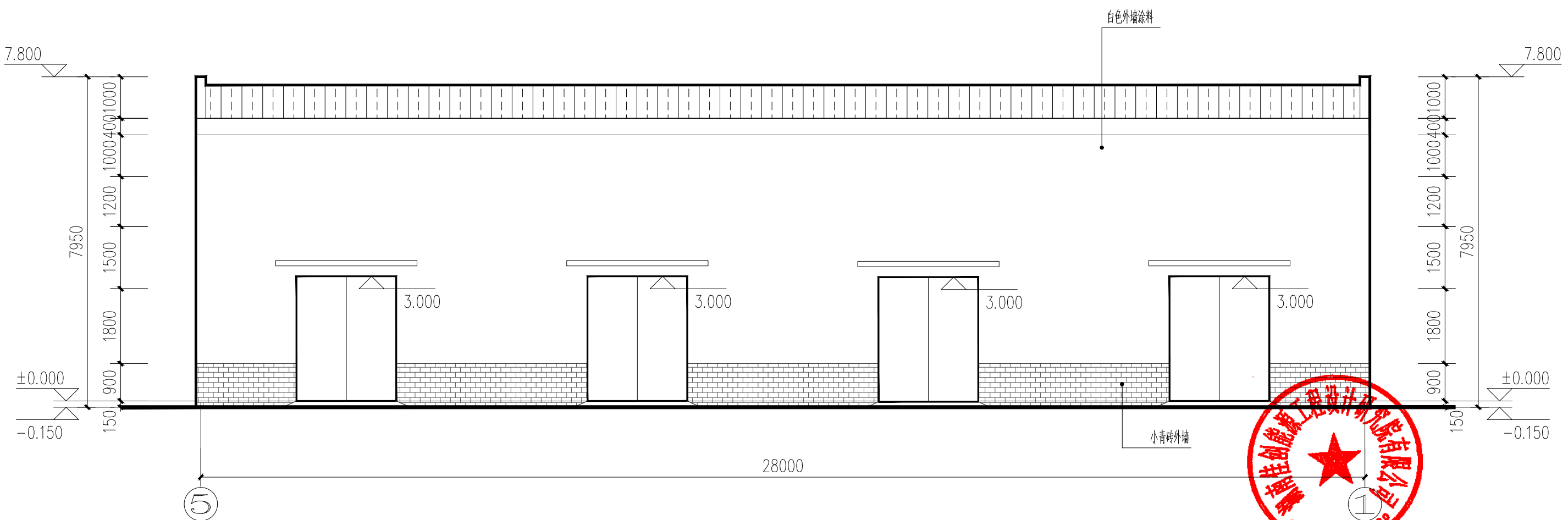
⑤ ~ ① 轴立面图
