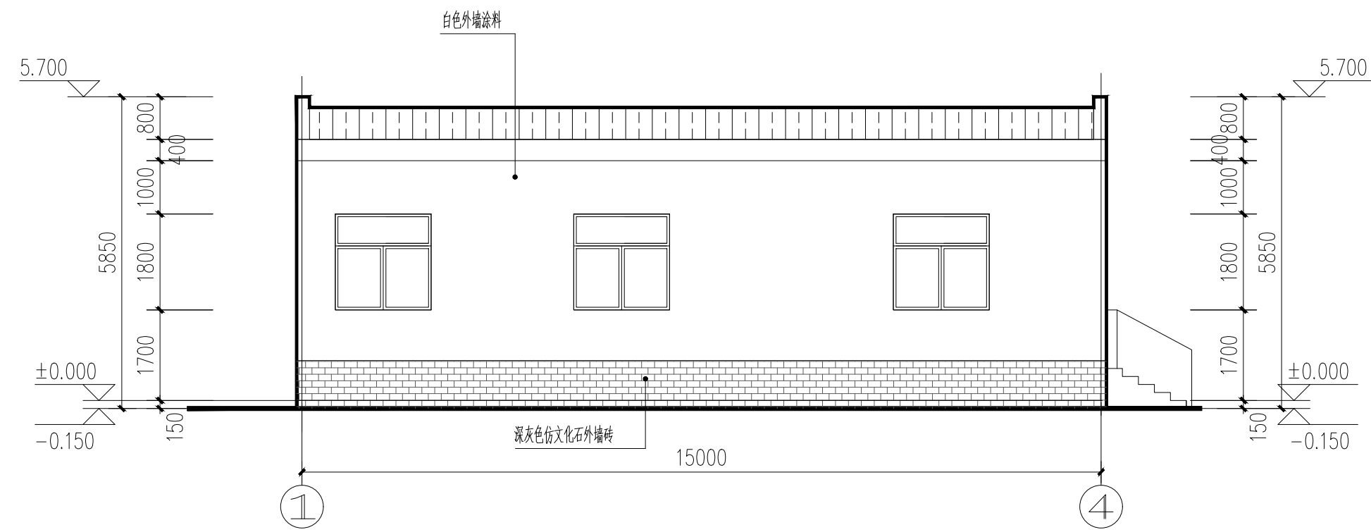
1~4 轴立面图 1:100
