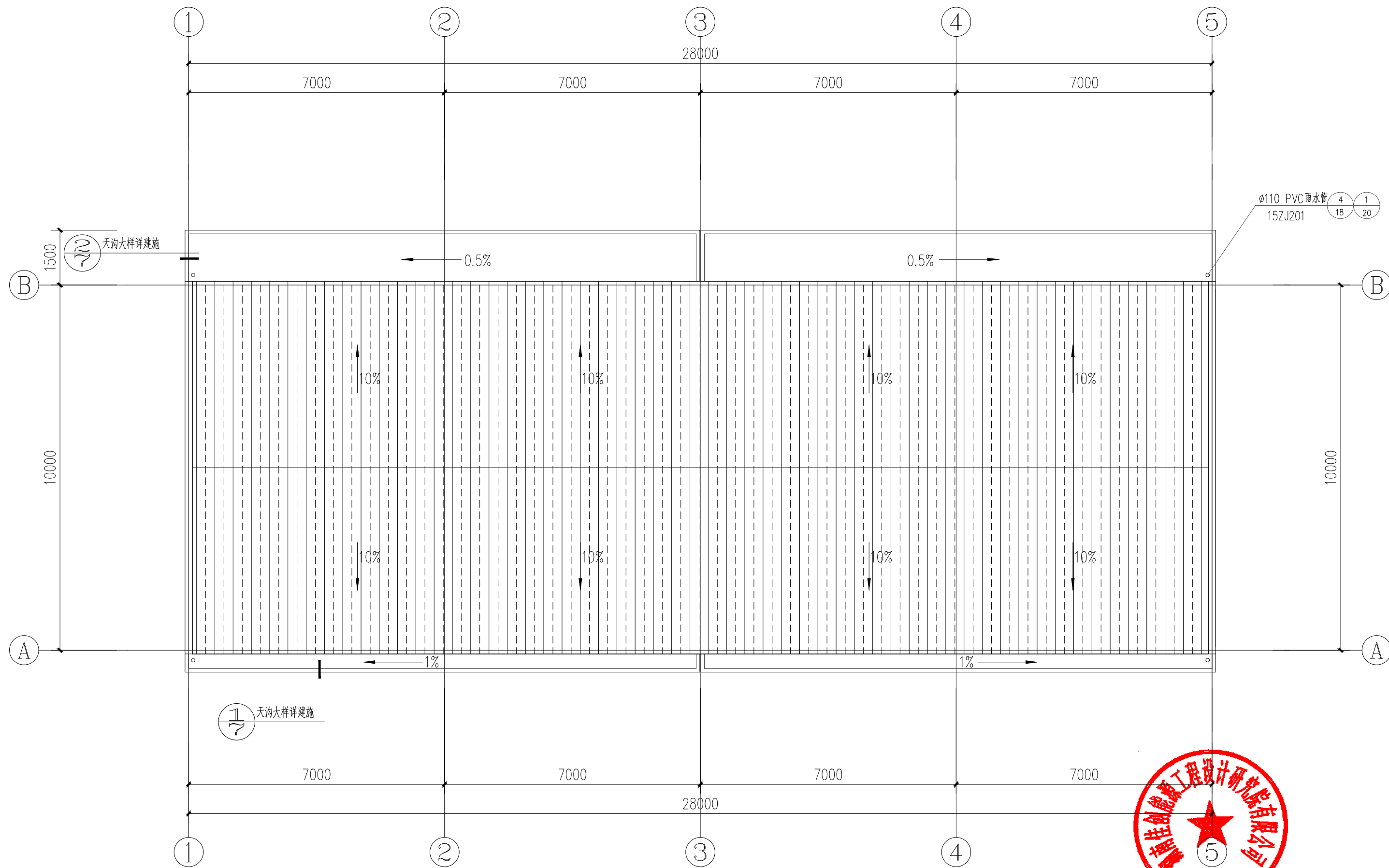
屋顶平面图 1:100
