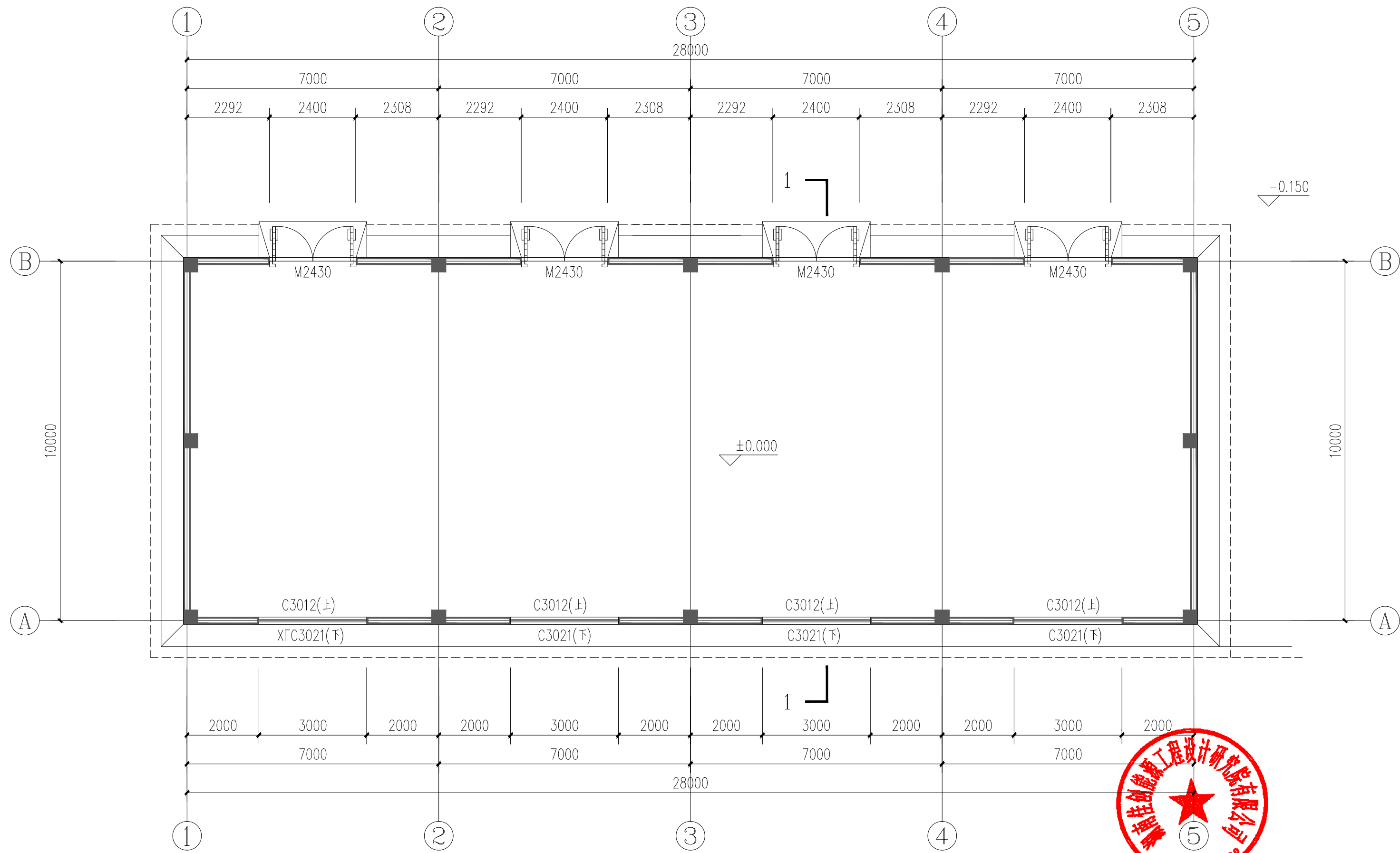
一层平面图 1: 100 本层建筑面积: 287.64m 2
