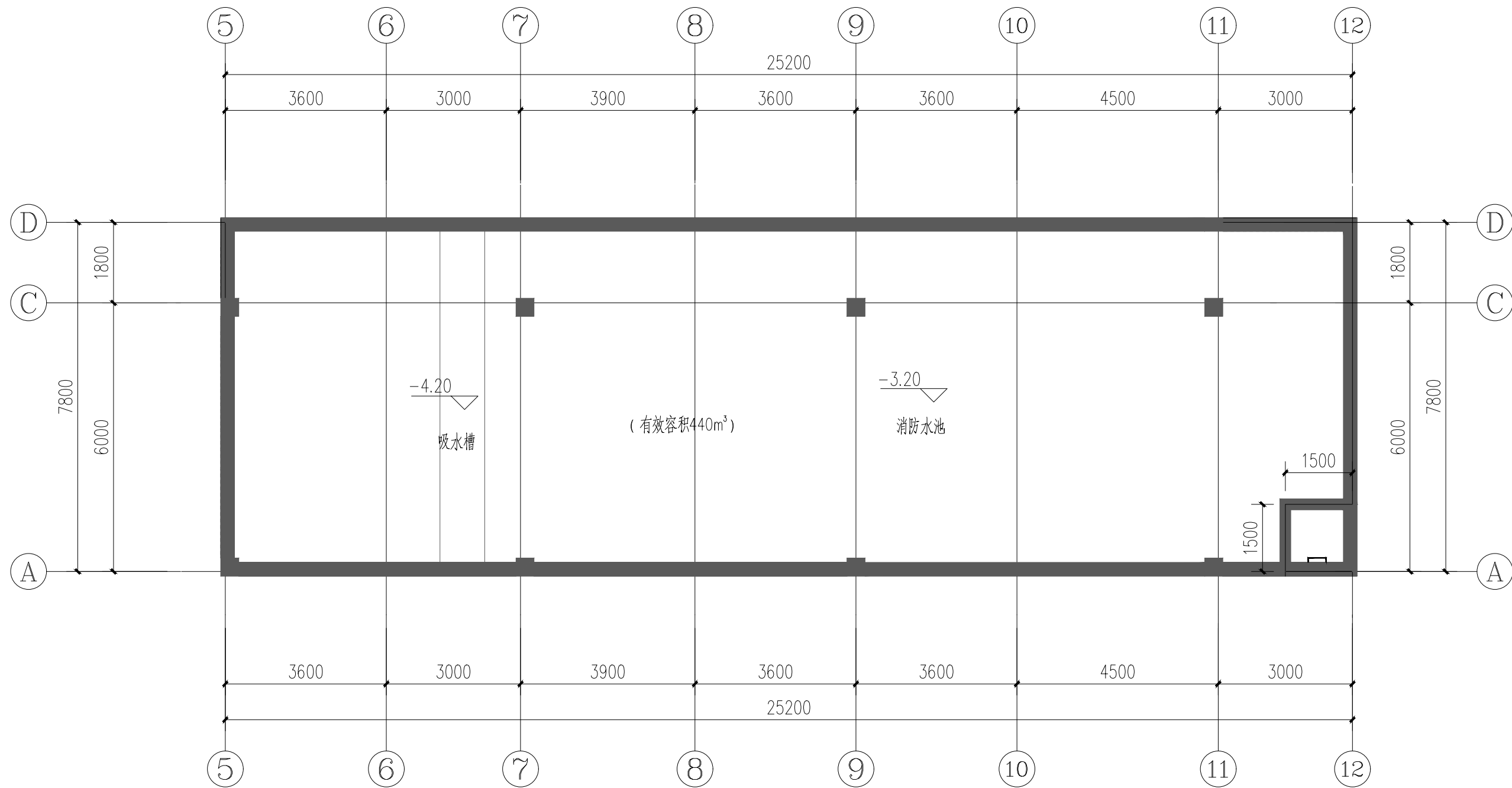
负一层平面图 1:100
