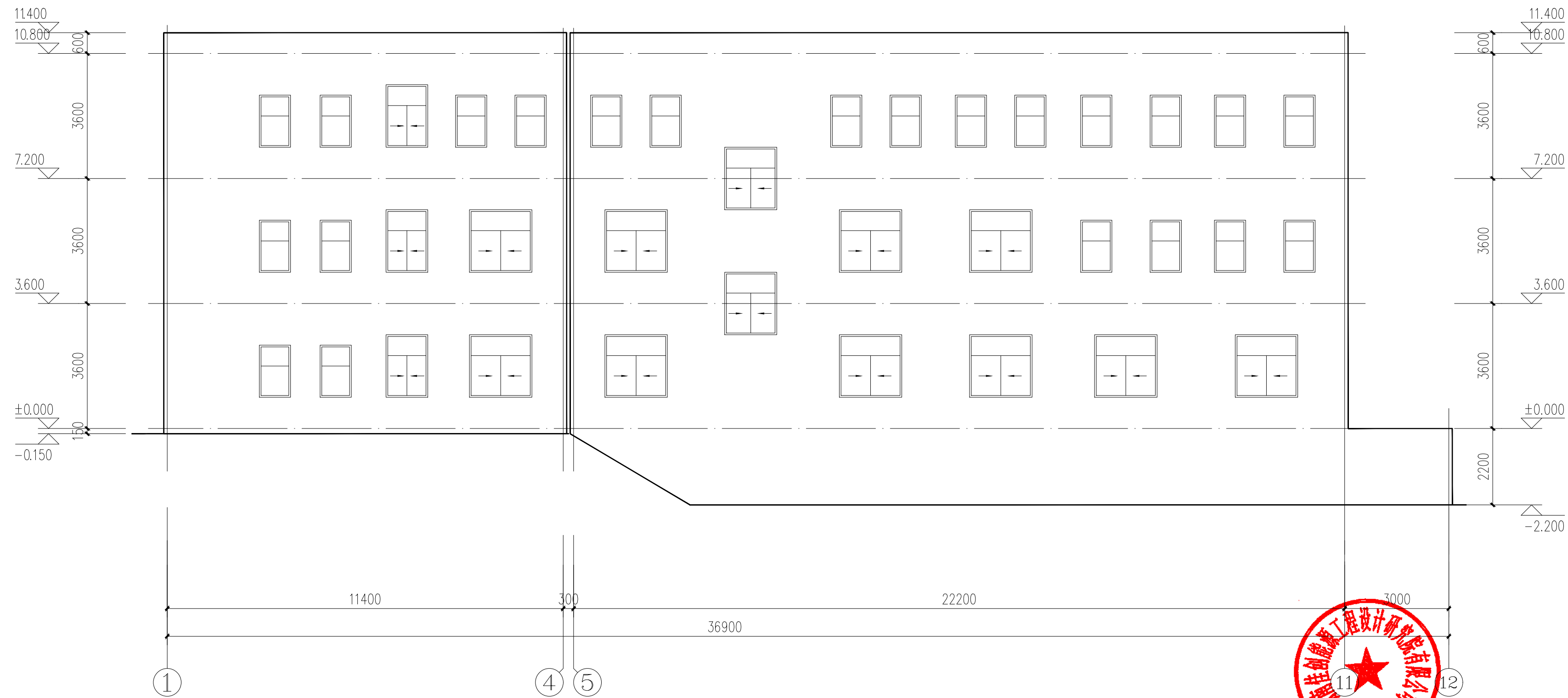
①~⑫轴立面图 1:100
