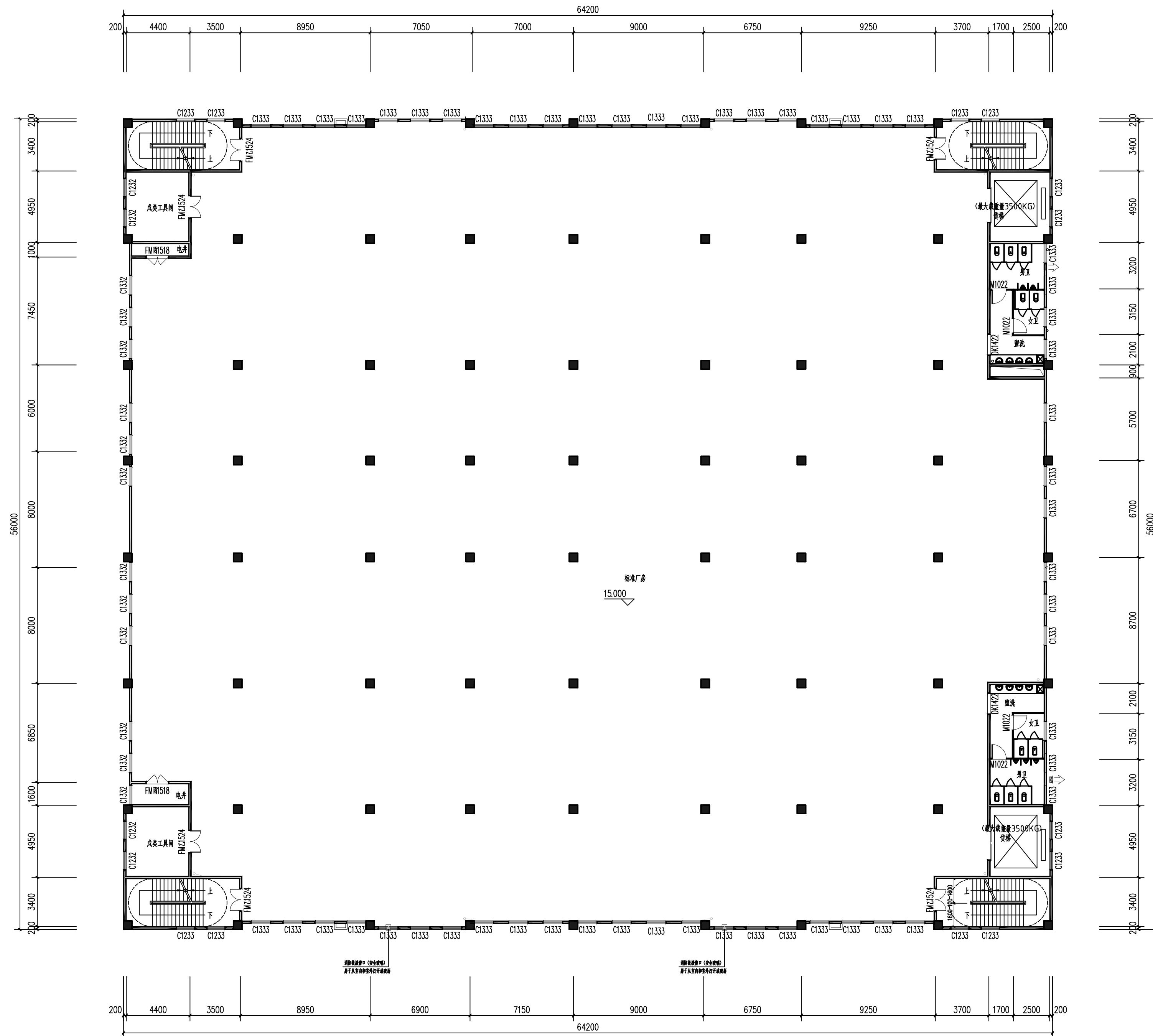
1:100 四层平面图 四层建筑面积: 3562.77m 2
