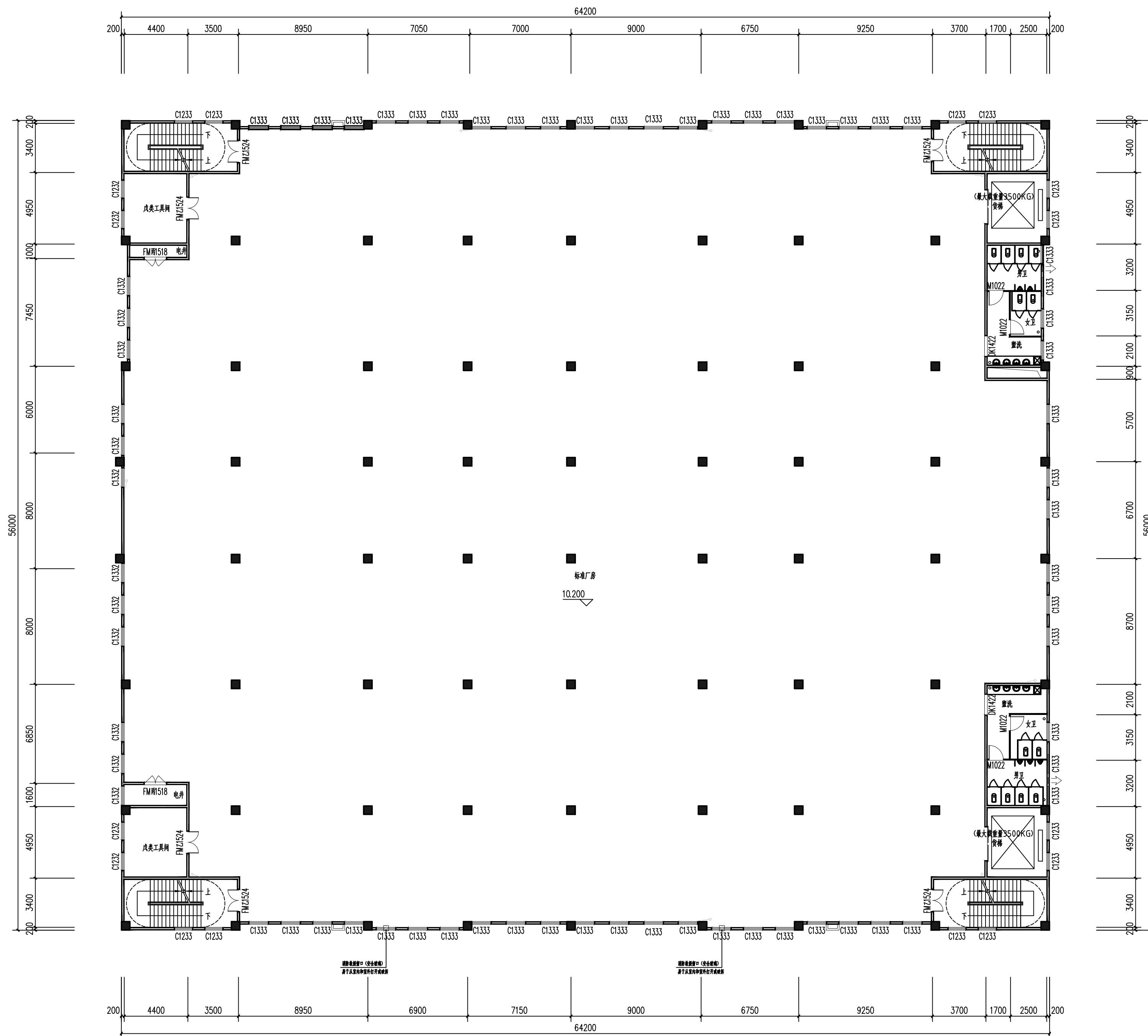
1:100 三层平面图 三层建筑面积: 3562.77m 2
