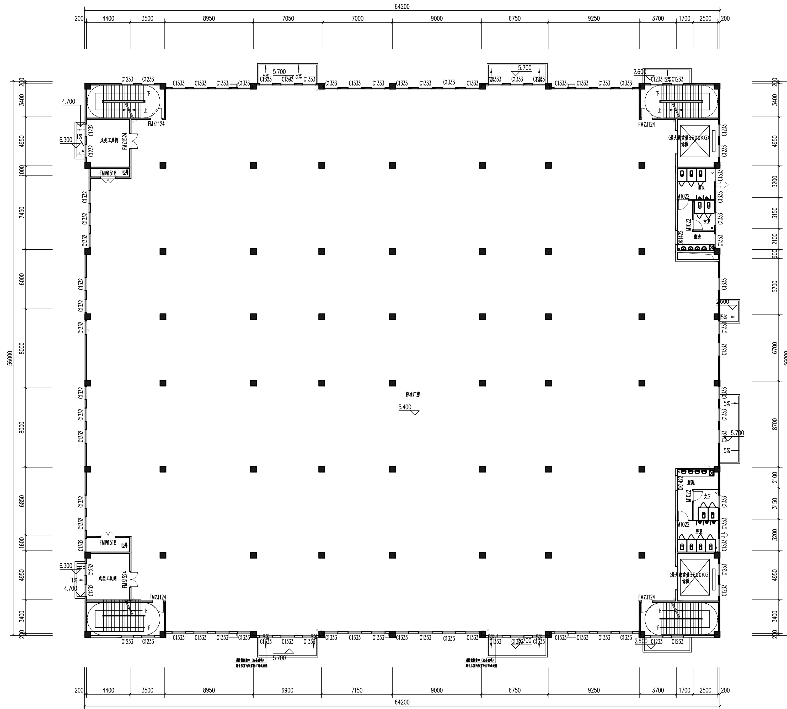
1:100 二层平面图 二层建筑面积: 3562.77m 2
